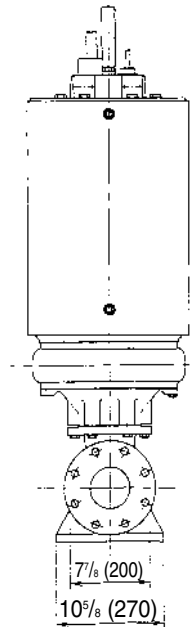
Flange (ANSI 125 PSI F.F)
